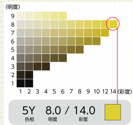
等色相面（5Y）の明度と彩度
