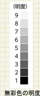
無彩色の明度
